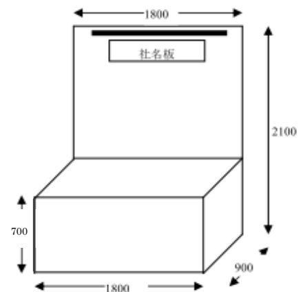
基礎小間姿図
